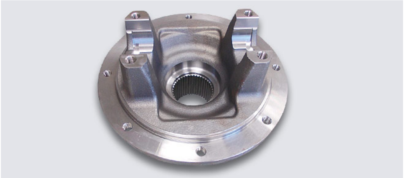
Flansch Half round yoke mit angegossener Bremsscheibe
